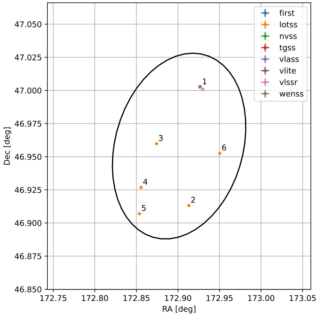
4FGL J1131.6+4657
