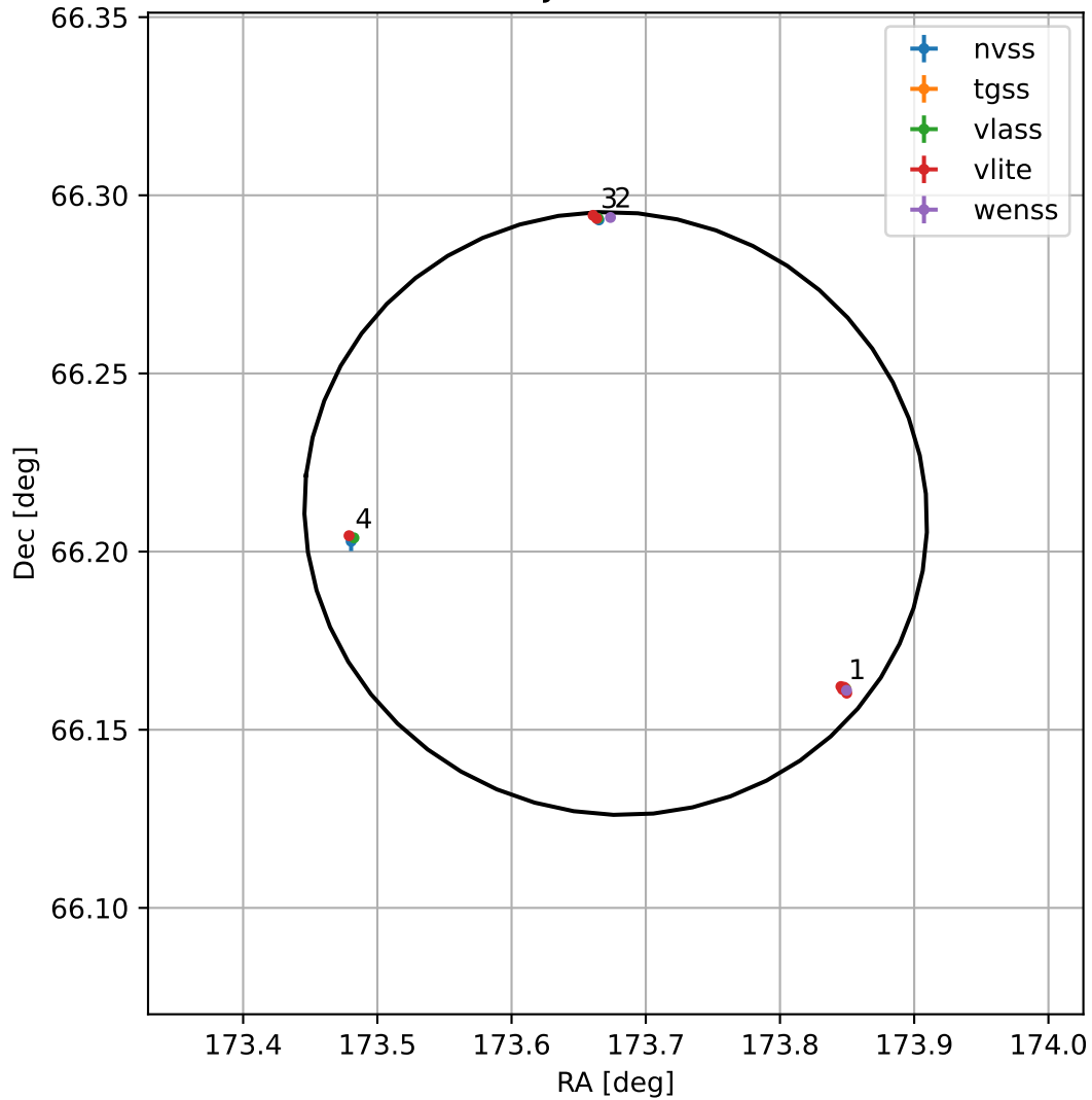
4FGL J1134.7+6612
