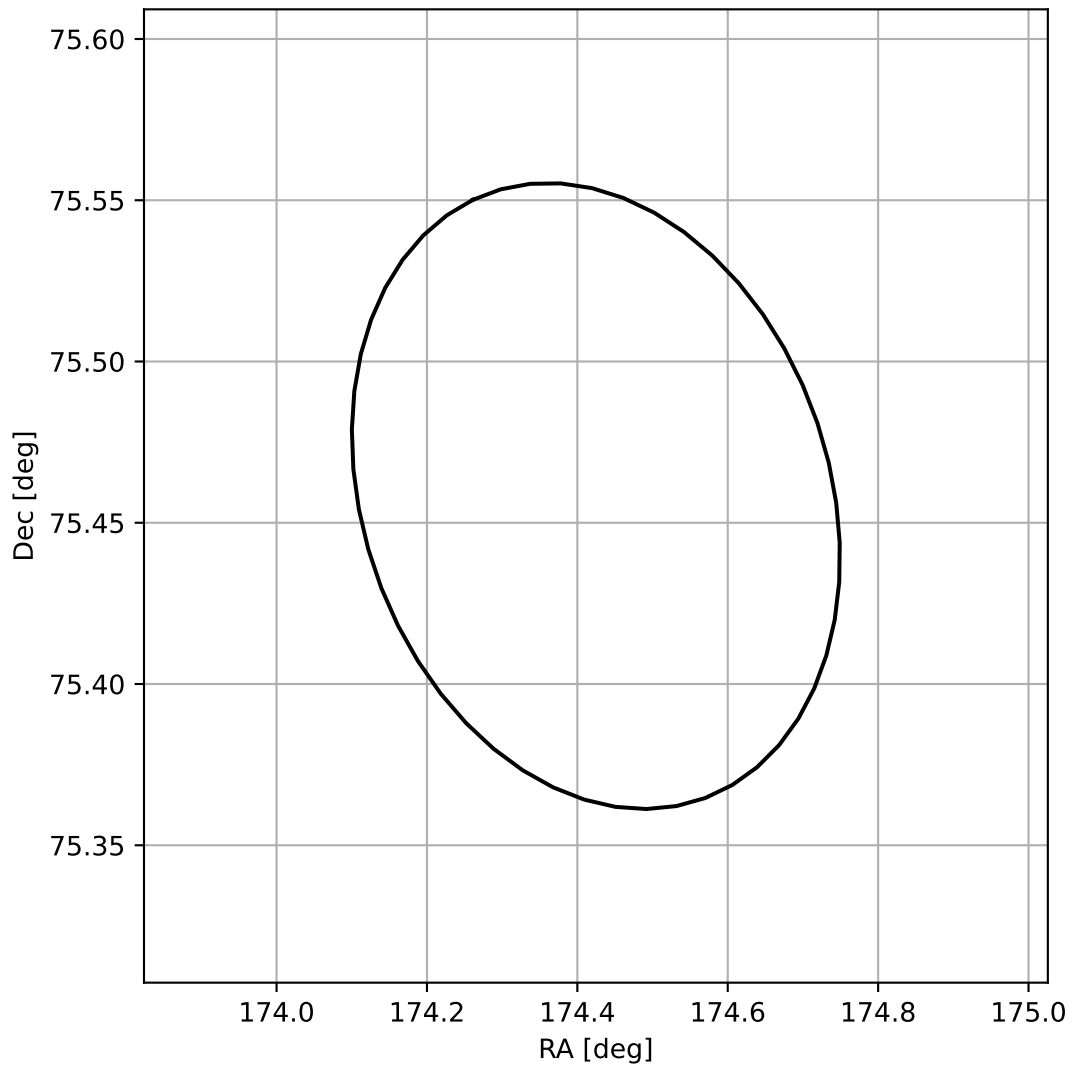
4FGL J1137.6+7527
