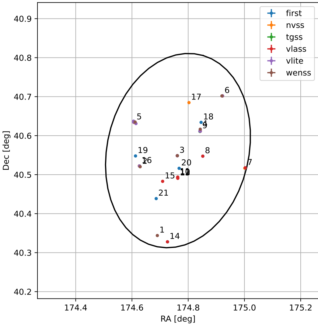
4FGL J1139.0+4033
