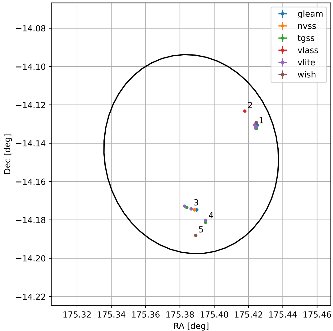
4FGL J1141.5-1408
