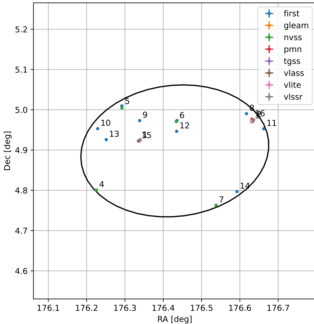
4FGL J1145.7+0453
