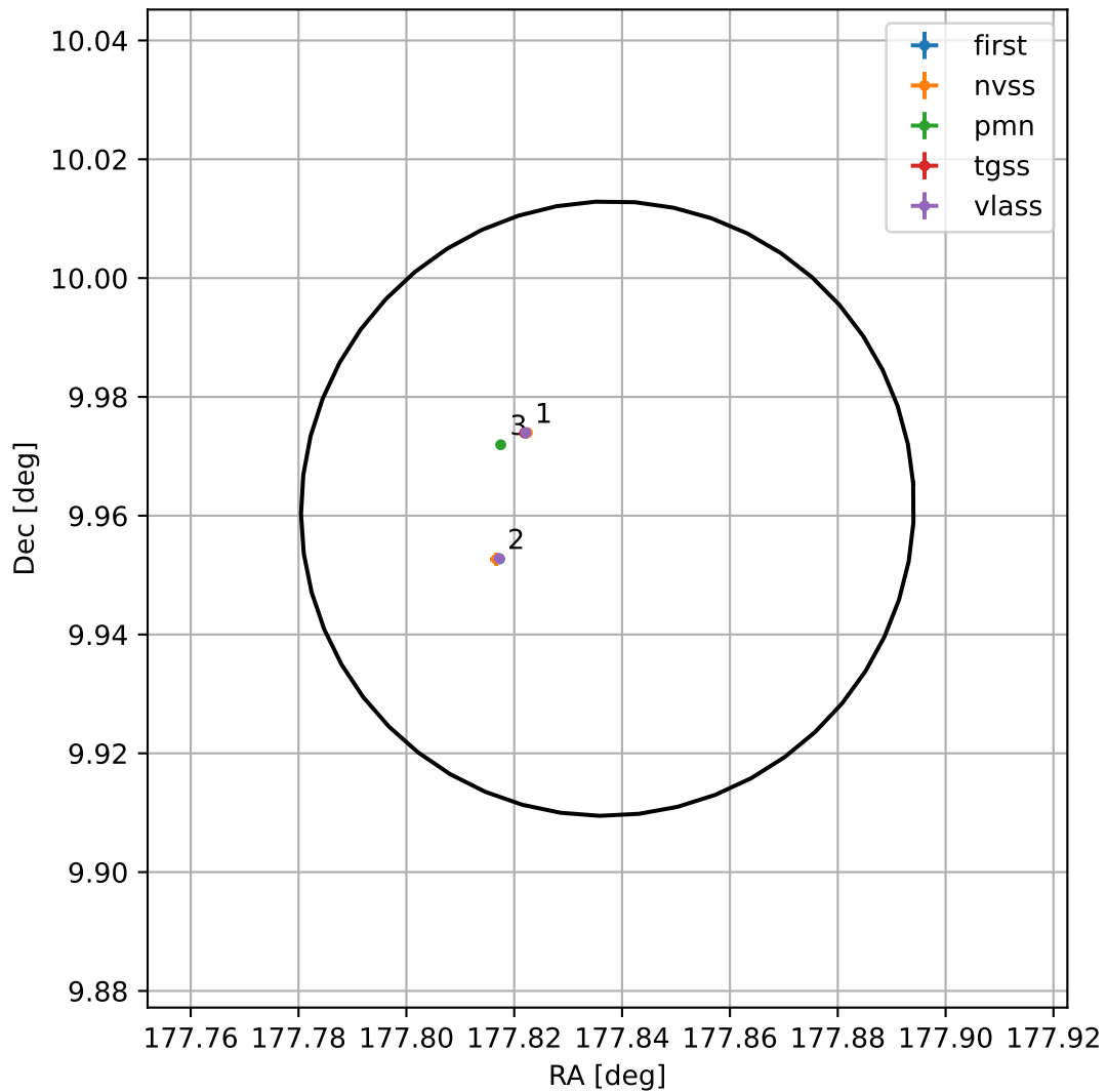
4FGL J1151.3+0957
