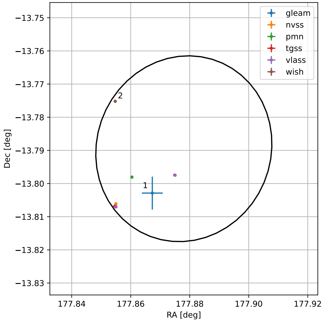
4FGL J1151.5-1347
