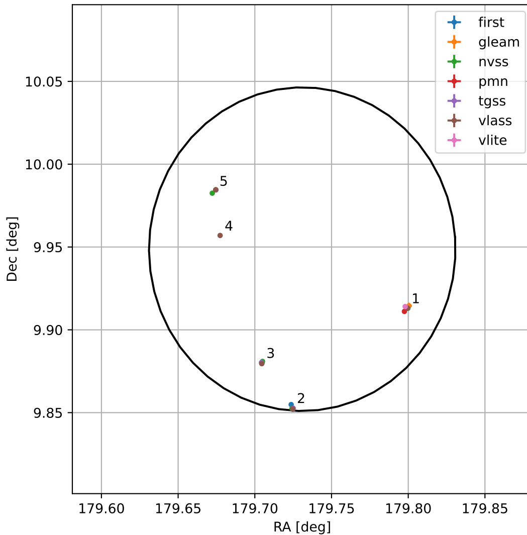
4FGL J1158.9+0956
