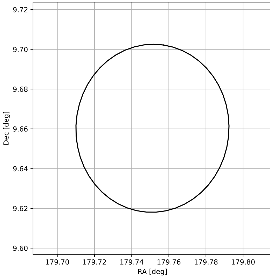
4FGL J1159.0+0939
