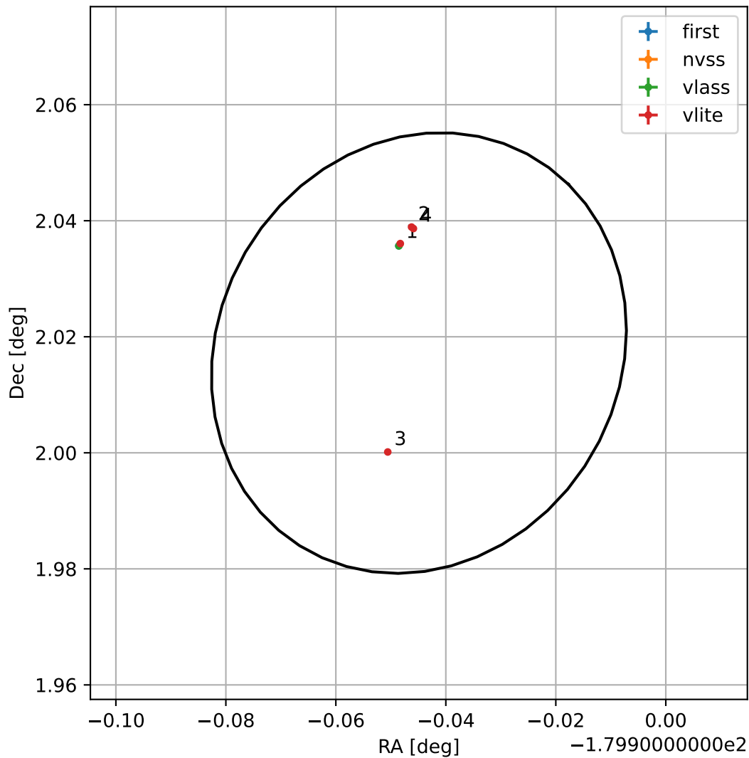
4FGL J1200.2+0201
