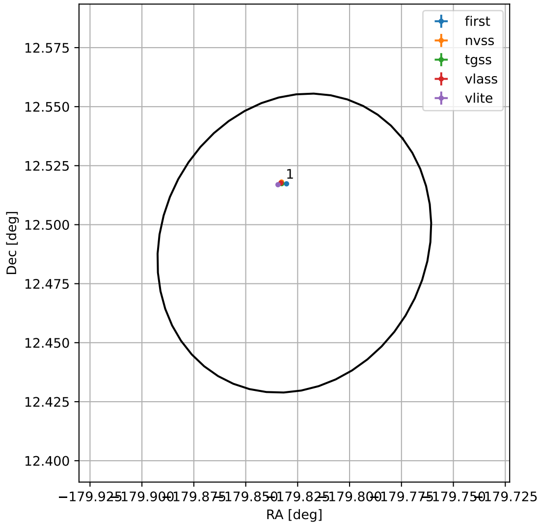
4FGL J1200.6+1229
