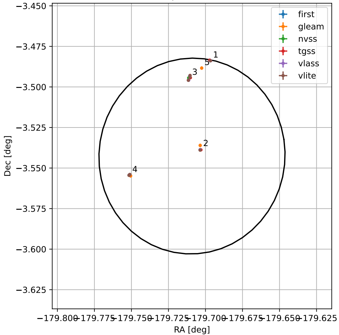
4FGL J1201.1-0332
