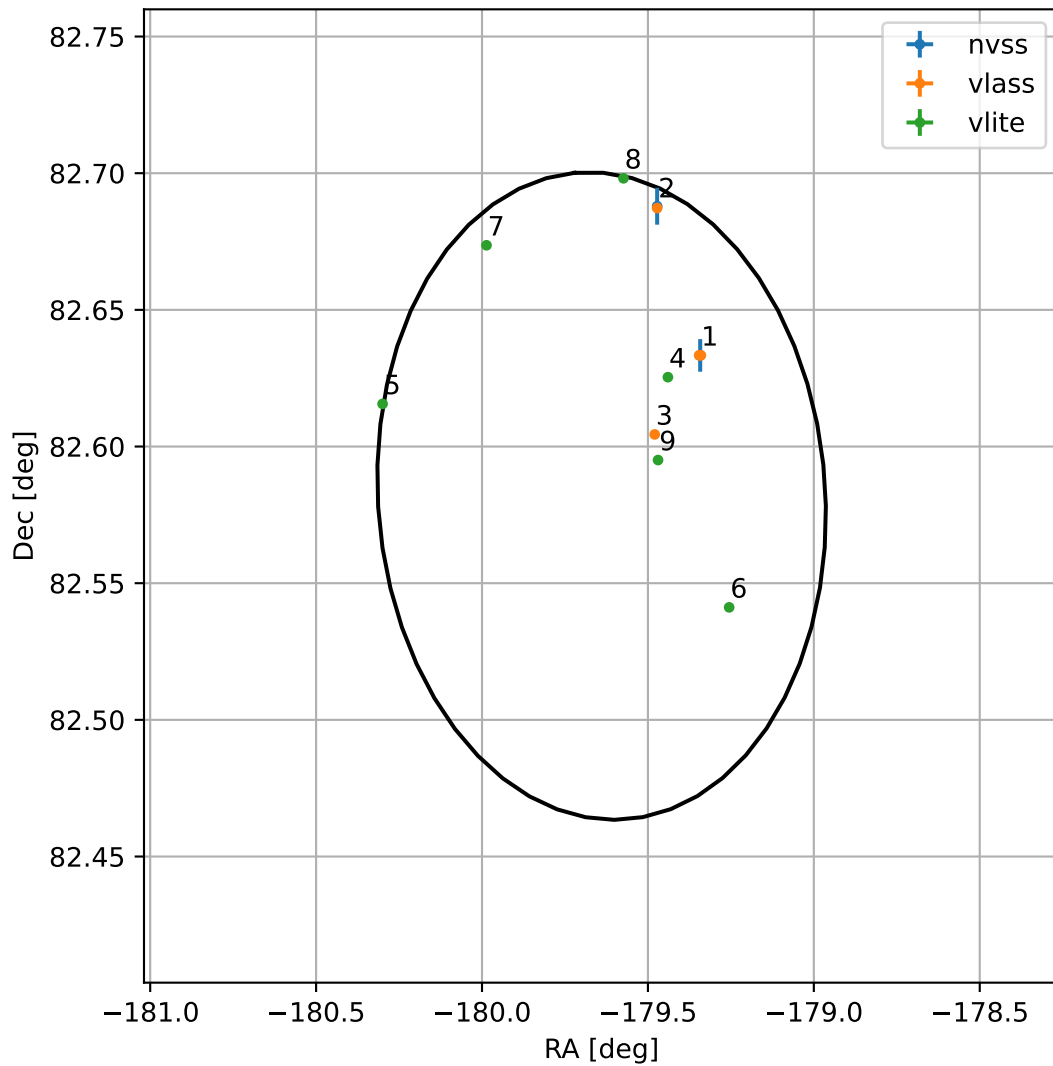
4FGL J1201.4+8234
