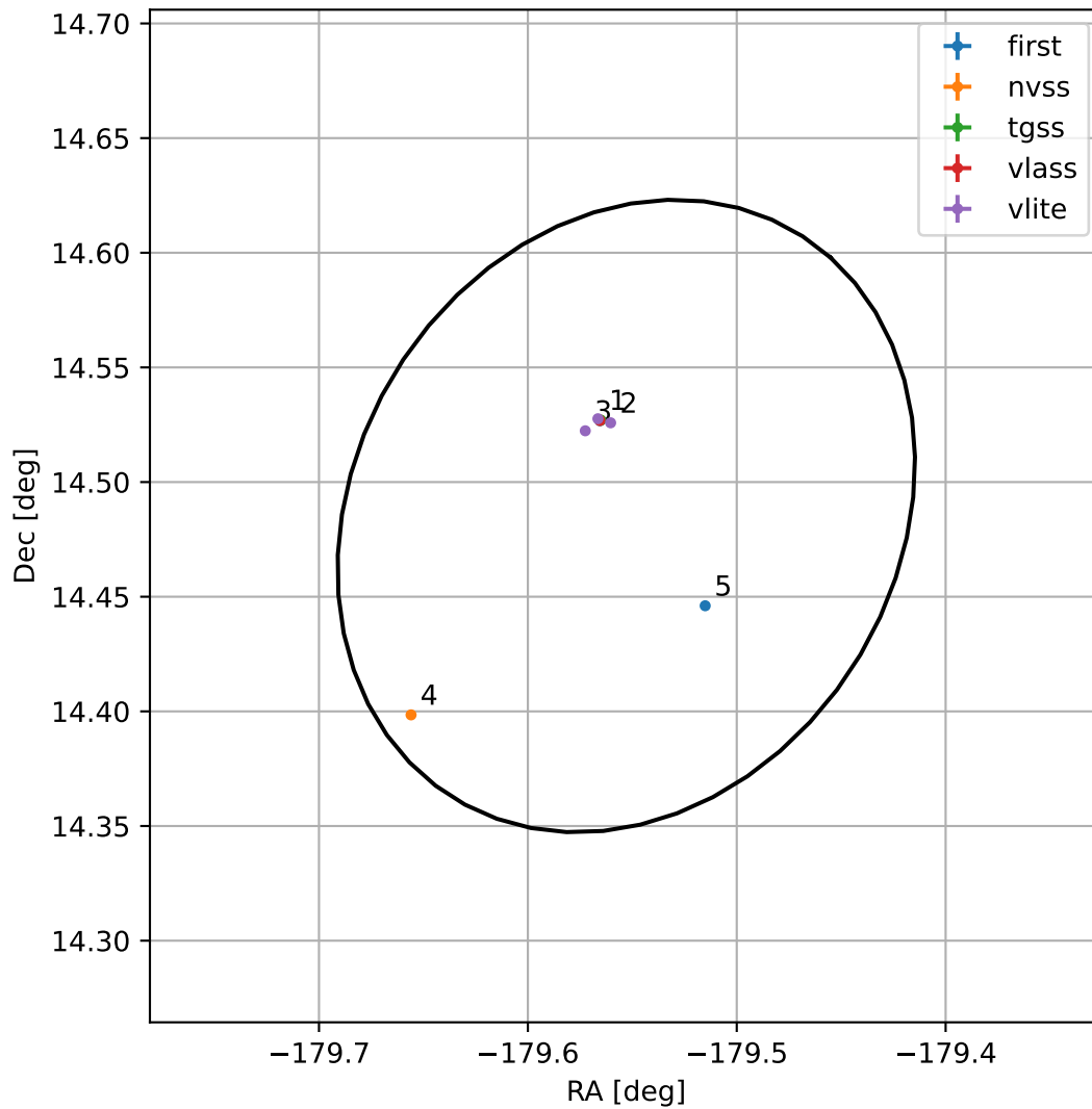
4FGL J1201.7+1429
