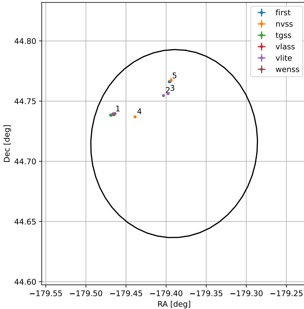
4FGL J1202.4+4442
