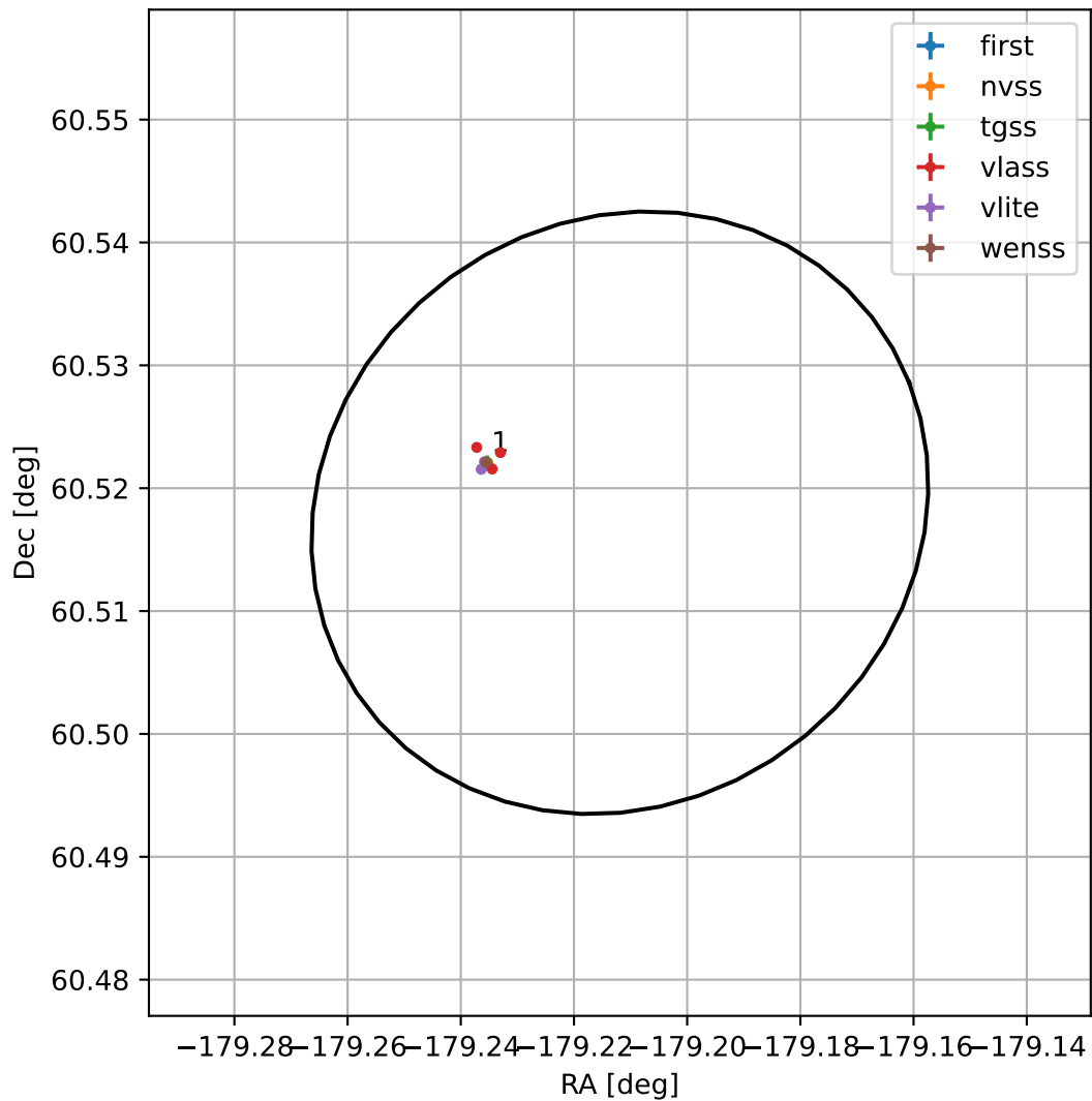
4FGL J1203.1+6031
