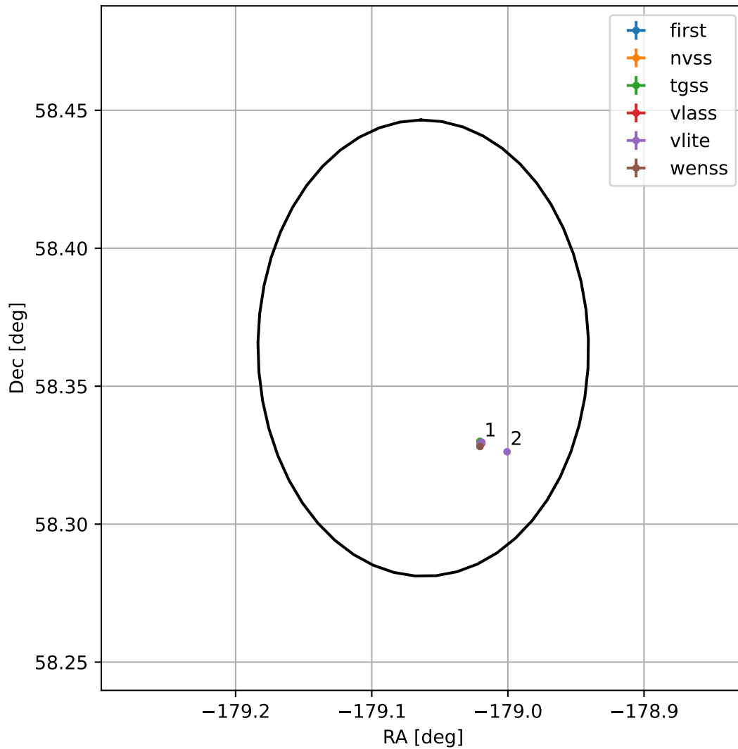
4FGL J1203.7+5821
