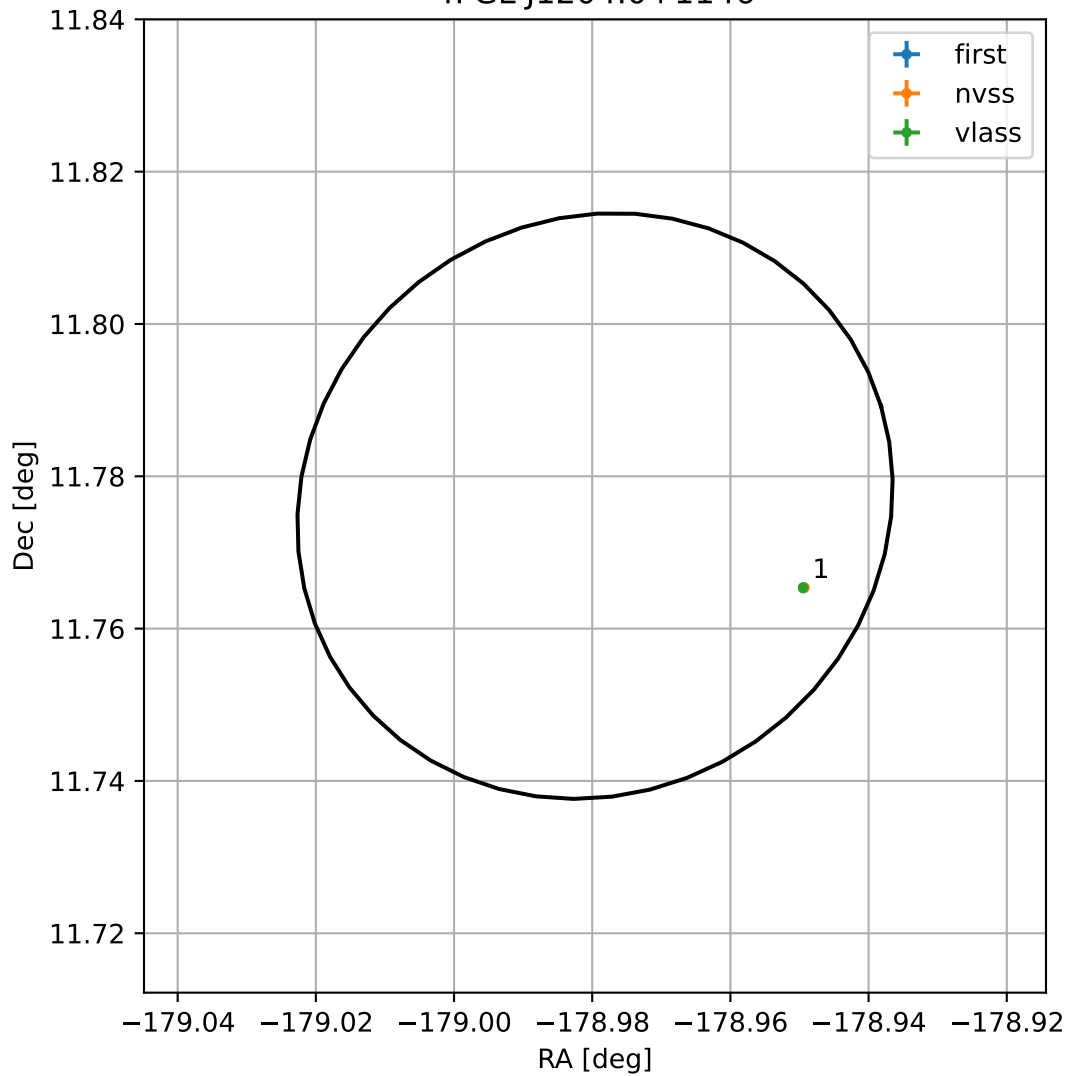
4FGL J1204.0+1146
