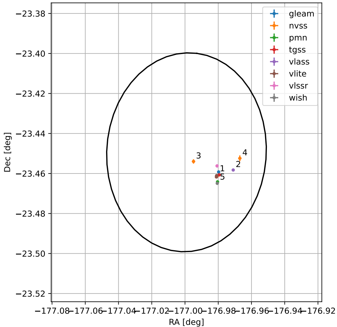
4FGL J1212.0-2326
