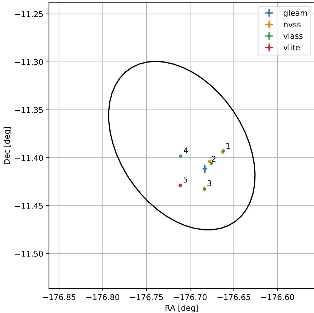
4FGL J1213.1-1123
