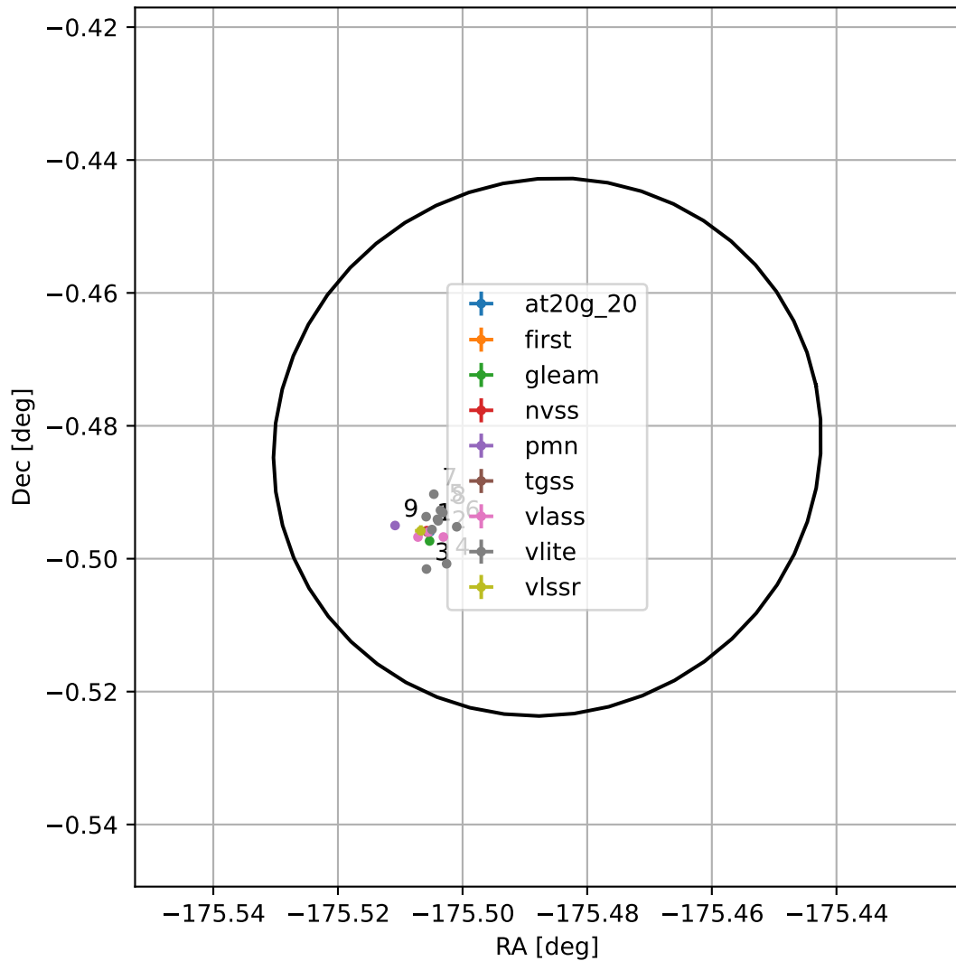
4FGL J1218.0-0028
