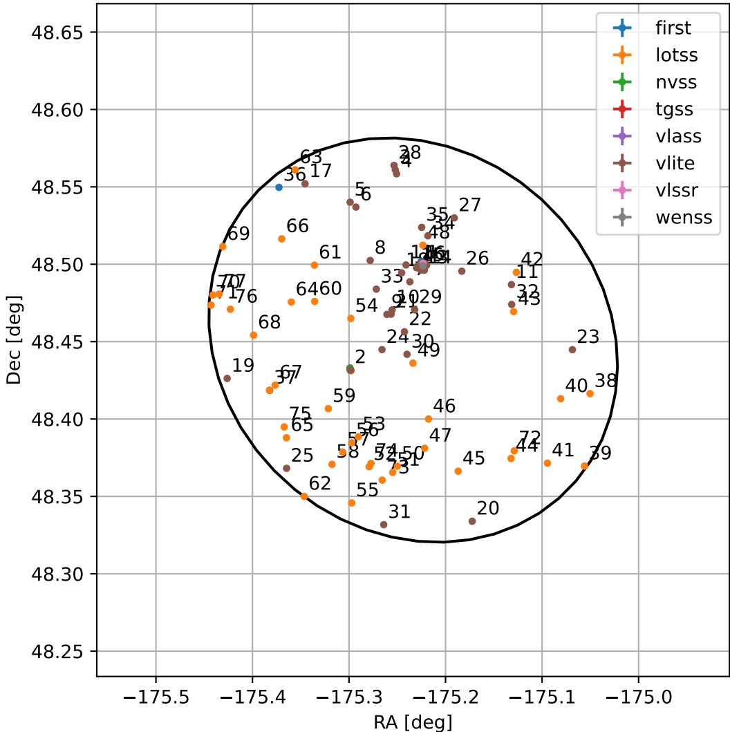
4FGL J1219.0+4827
