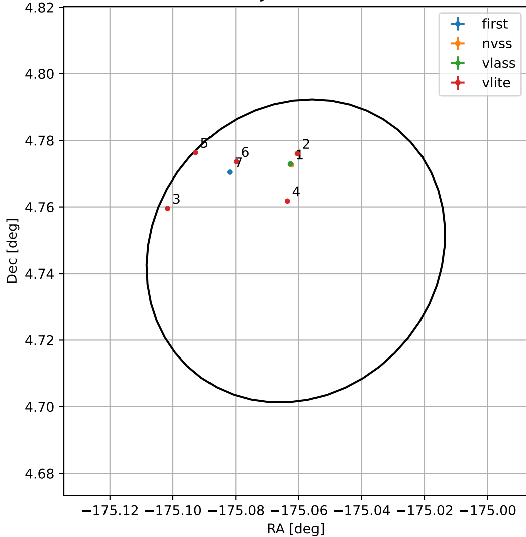
4FGL J1219.7+0444
