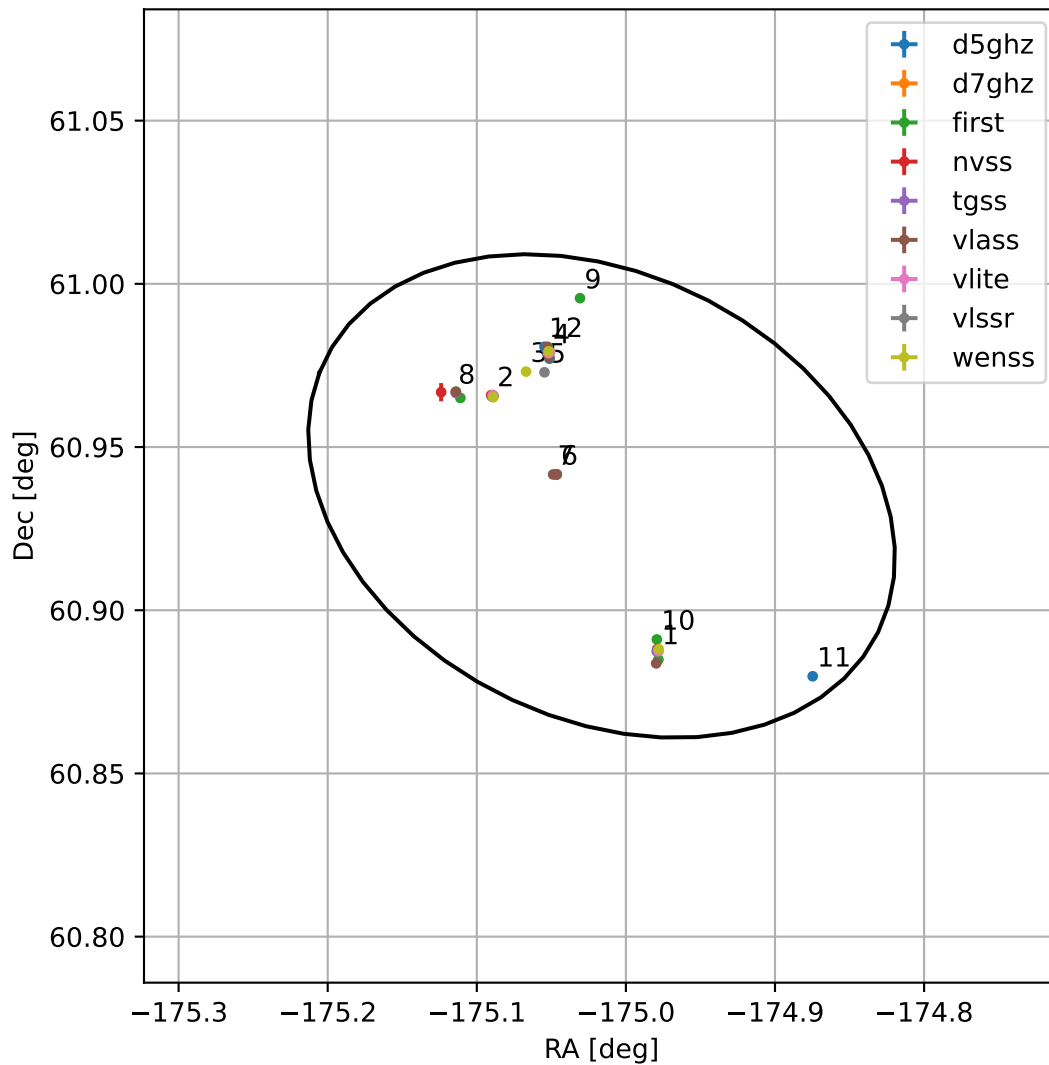
4FGL J1219.9+6056
