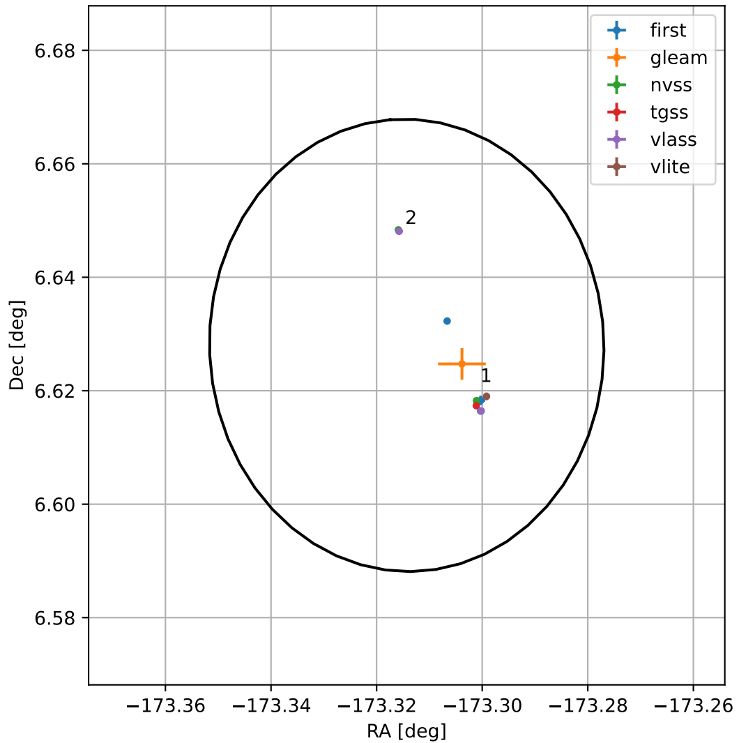
4FGL J1226.7+0637
