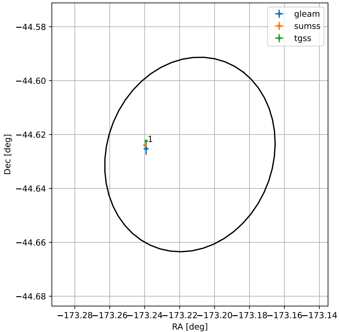
4FGL J1227.1-4437
