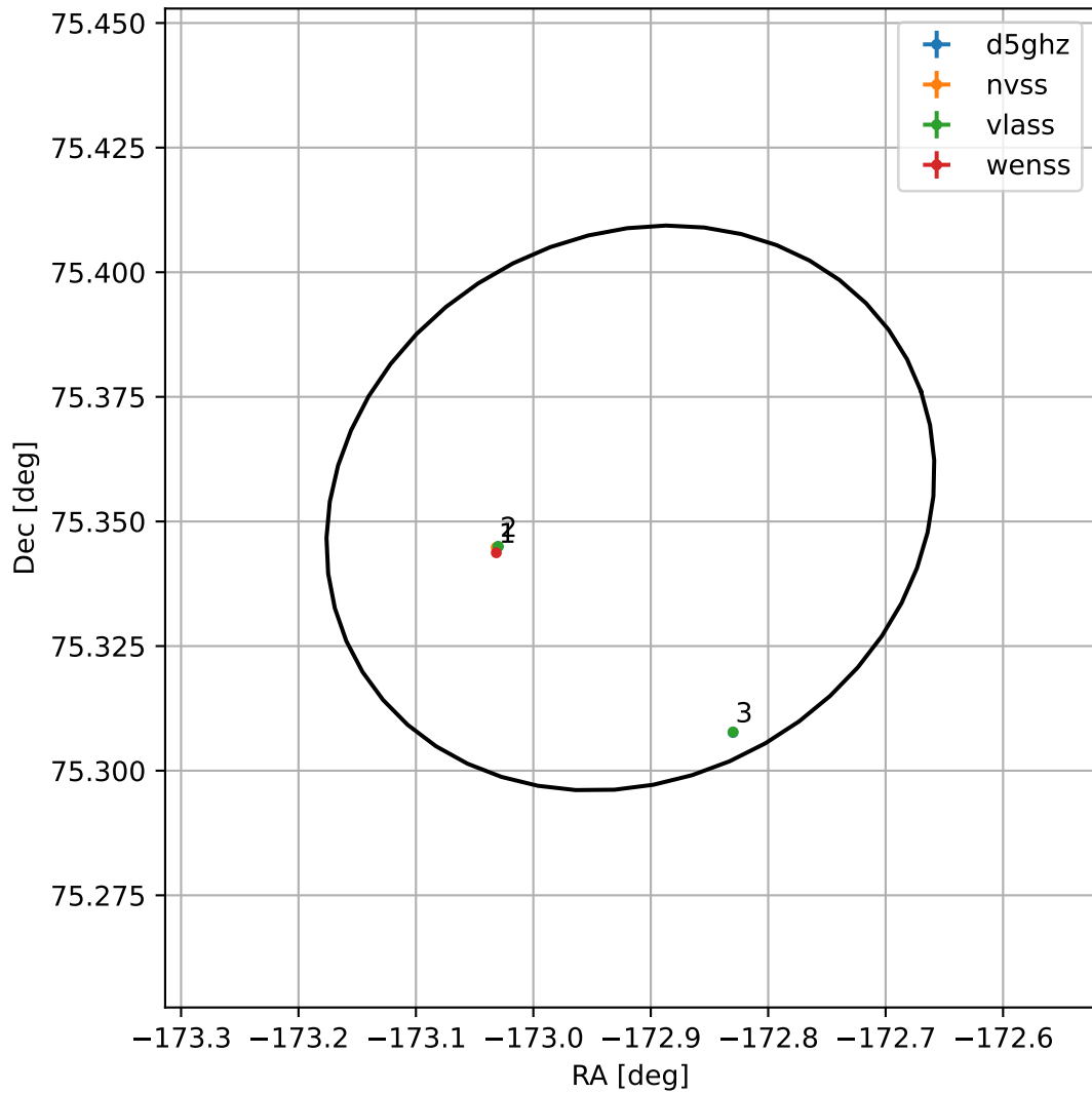
4FGL J1228.3+7521
