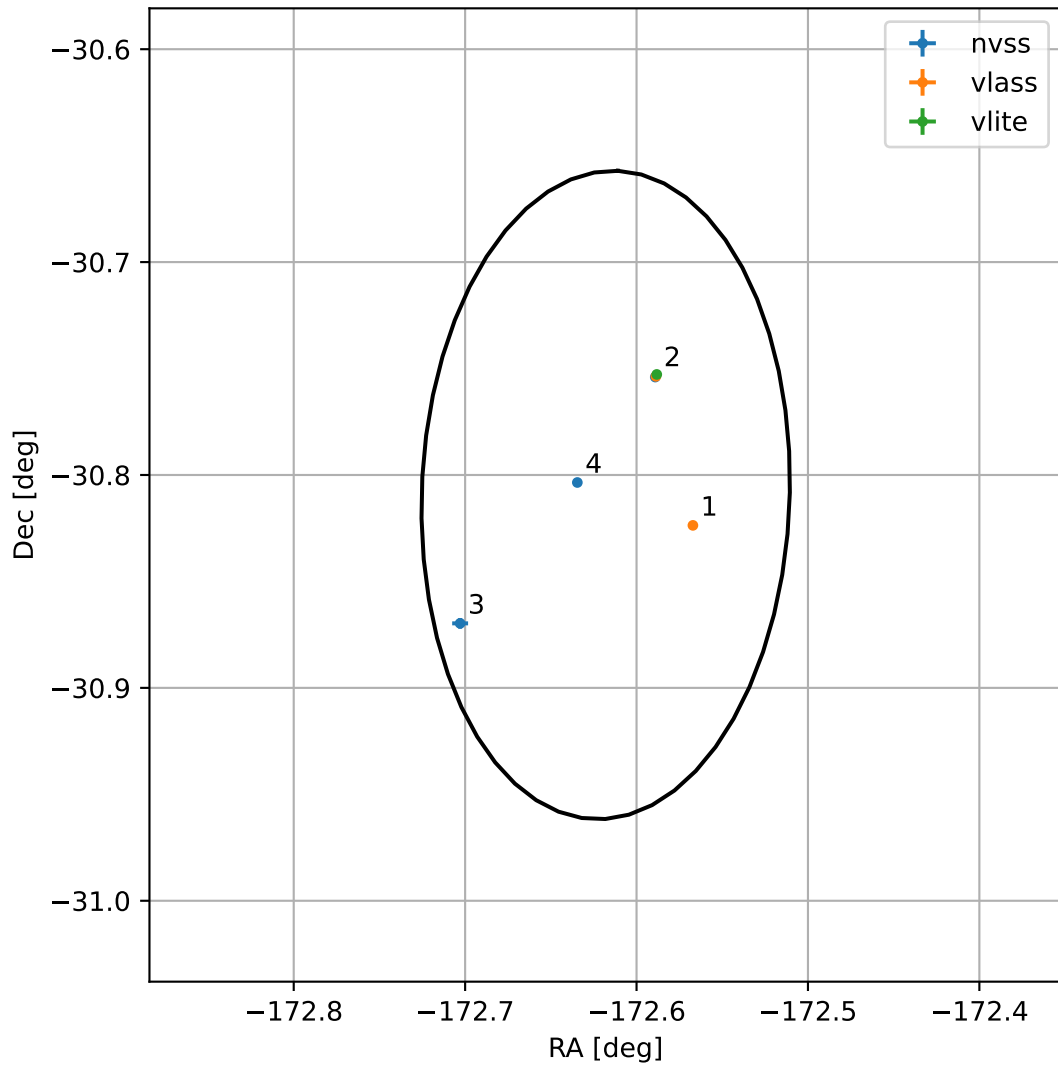
4FGL J1229.5-3048
