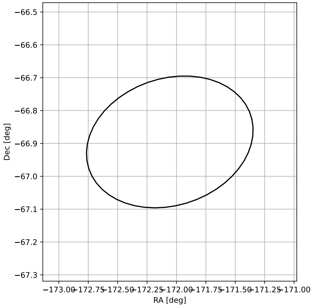
4FGL J1231.7-6653
