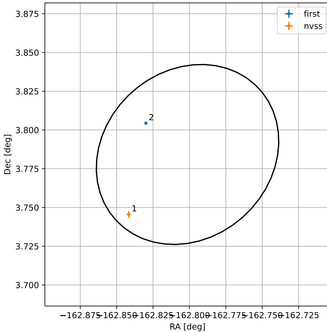
4FGL J1308.7+0347
