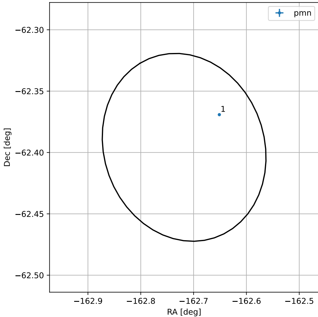
4FGL J1309.1-6223
