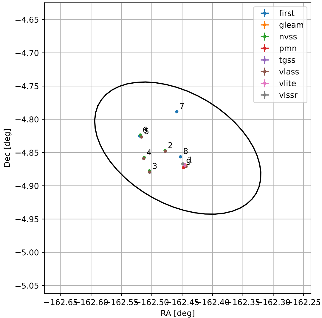
4FGL J1310.1-0450
