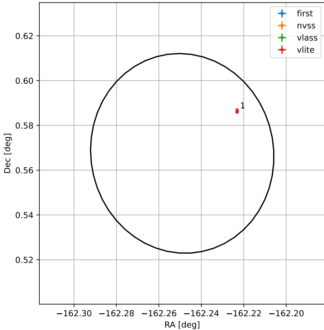
4FGL J1311.0+0034
