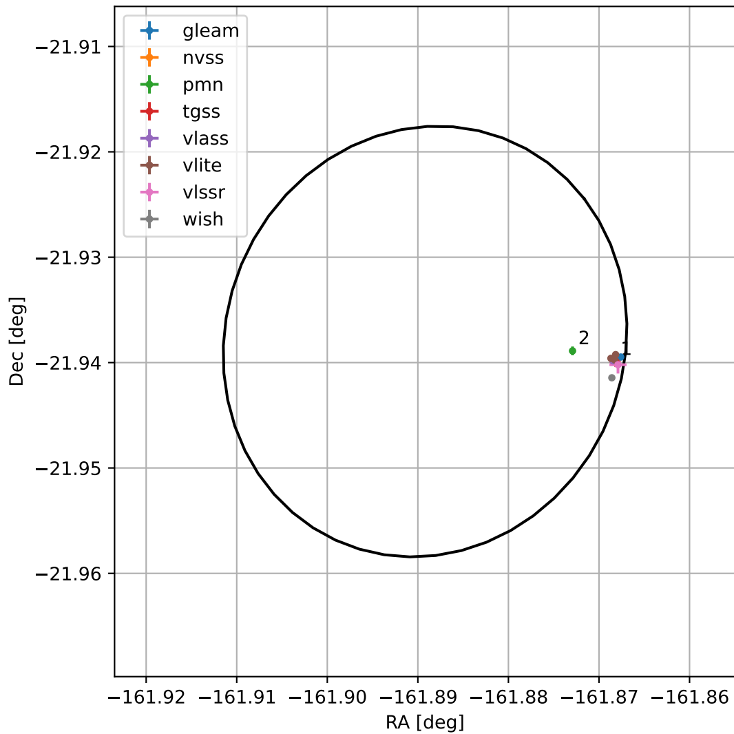
4FGL J1312.4-2156
