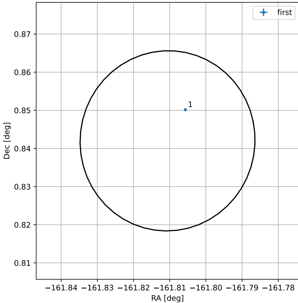
4FGL J1312.7+0050
