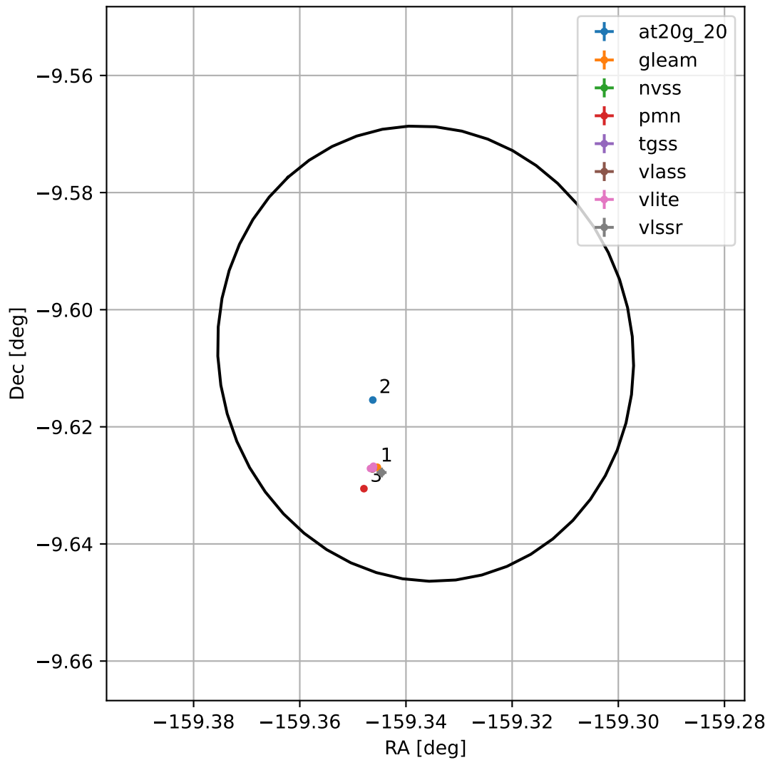
4FGL J1322.6-0936
