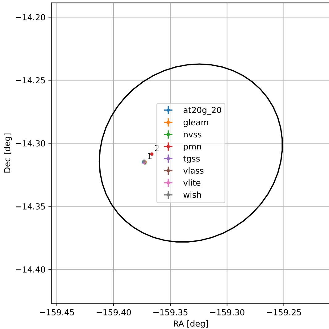
4FGL J1322.6-1418
