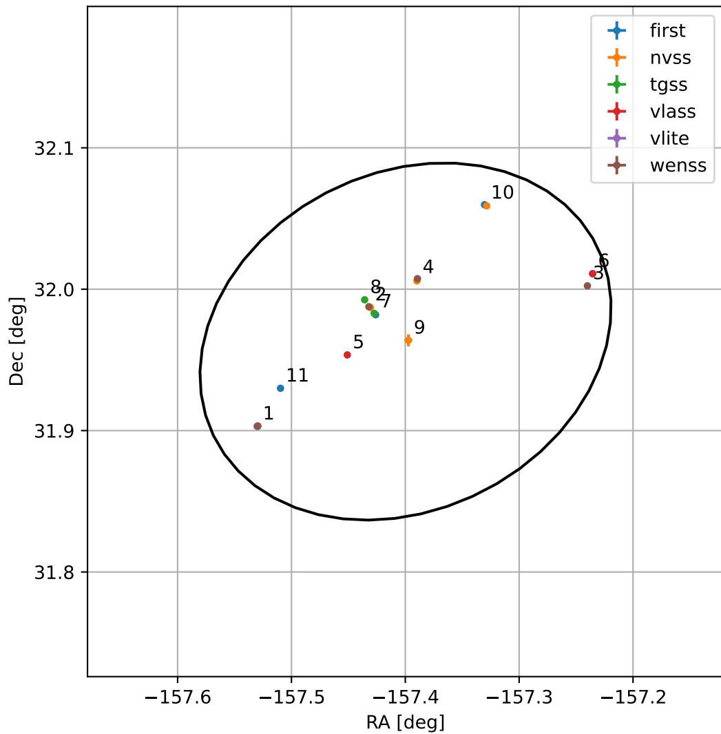
4FGL J1330.4+3157
