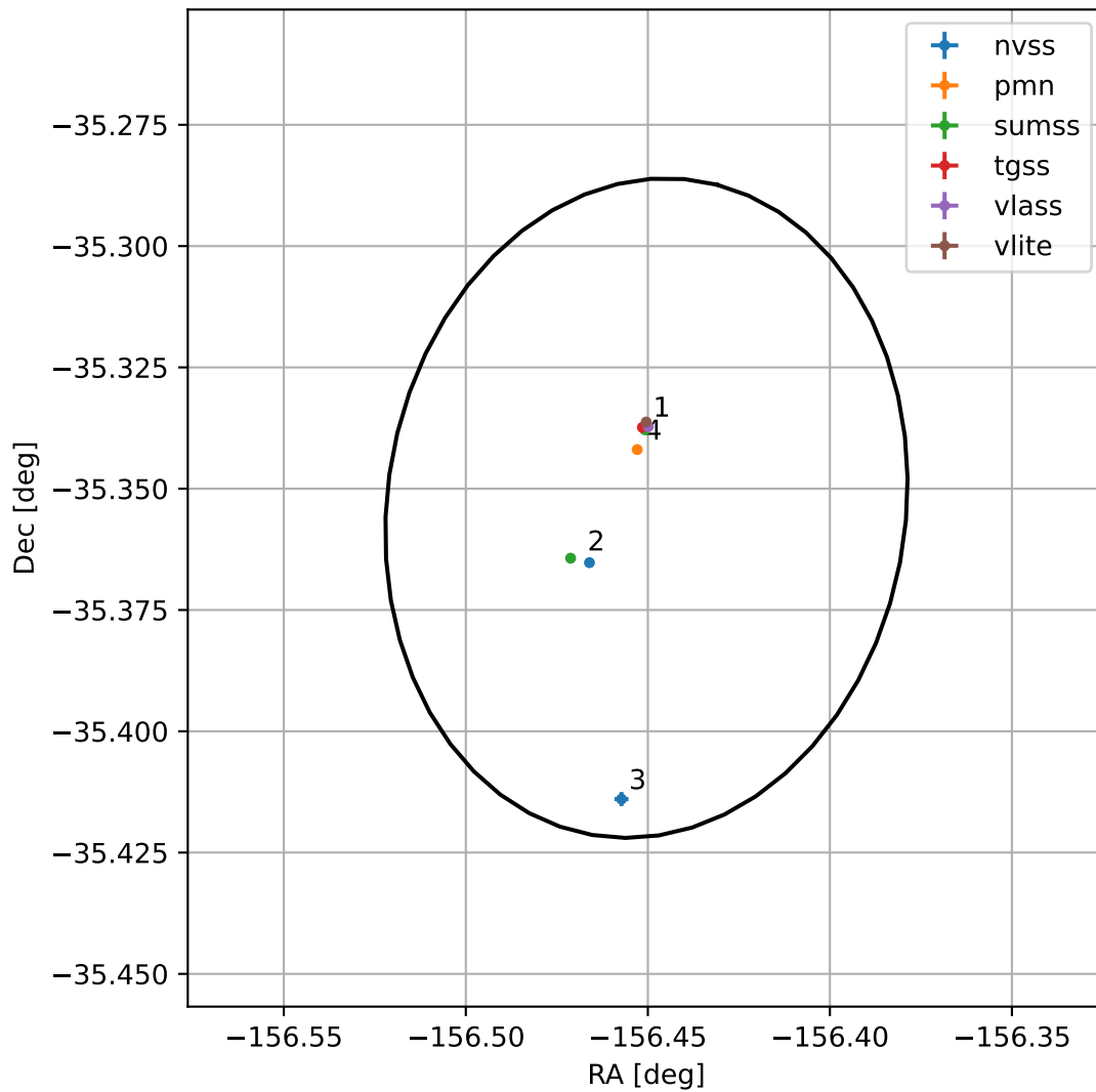
4FGL J1334.1-3521
