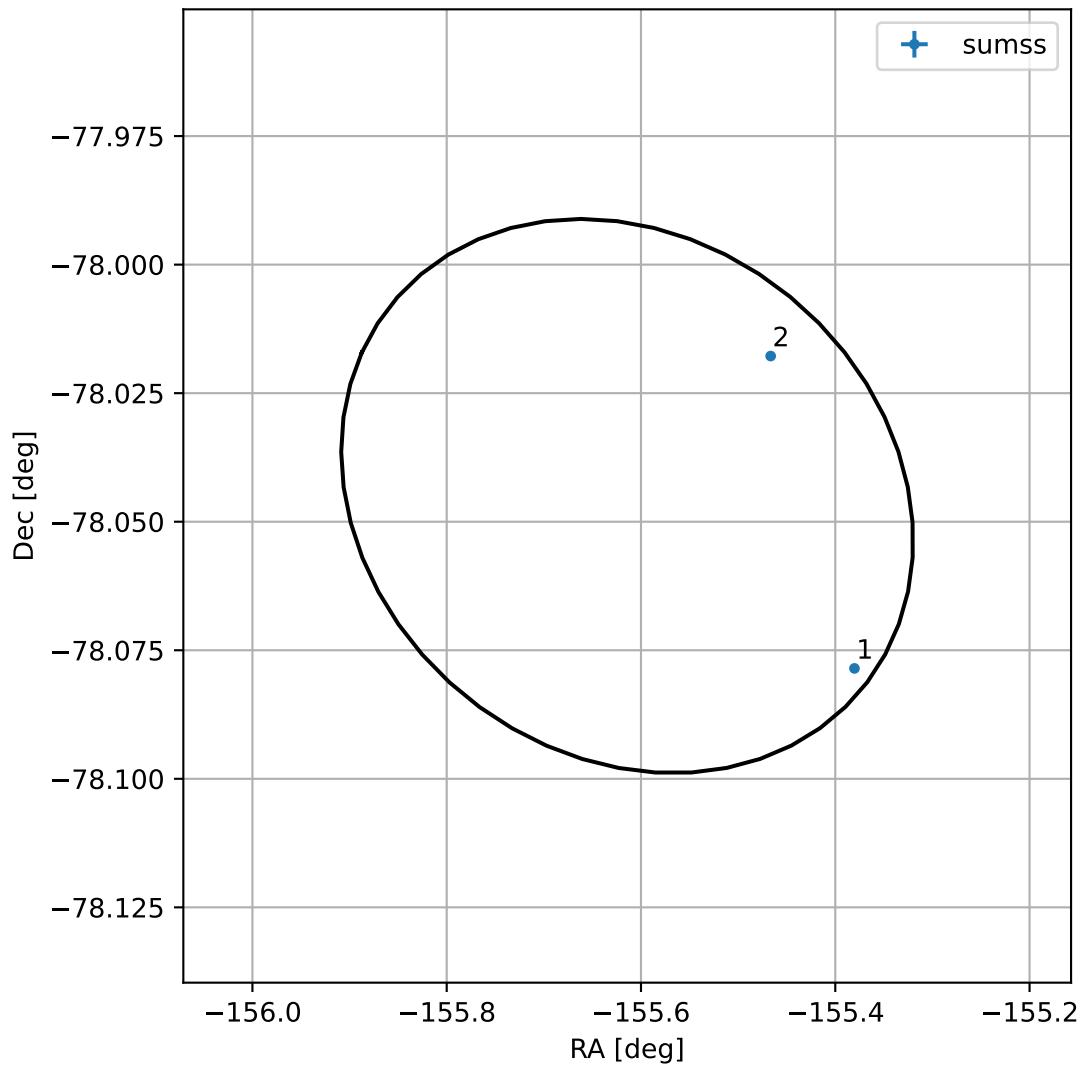
4FGL J1337.5-7802
