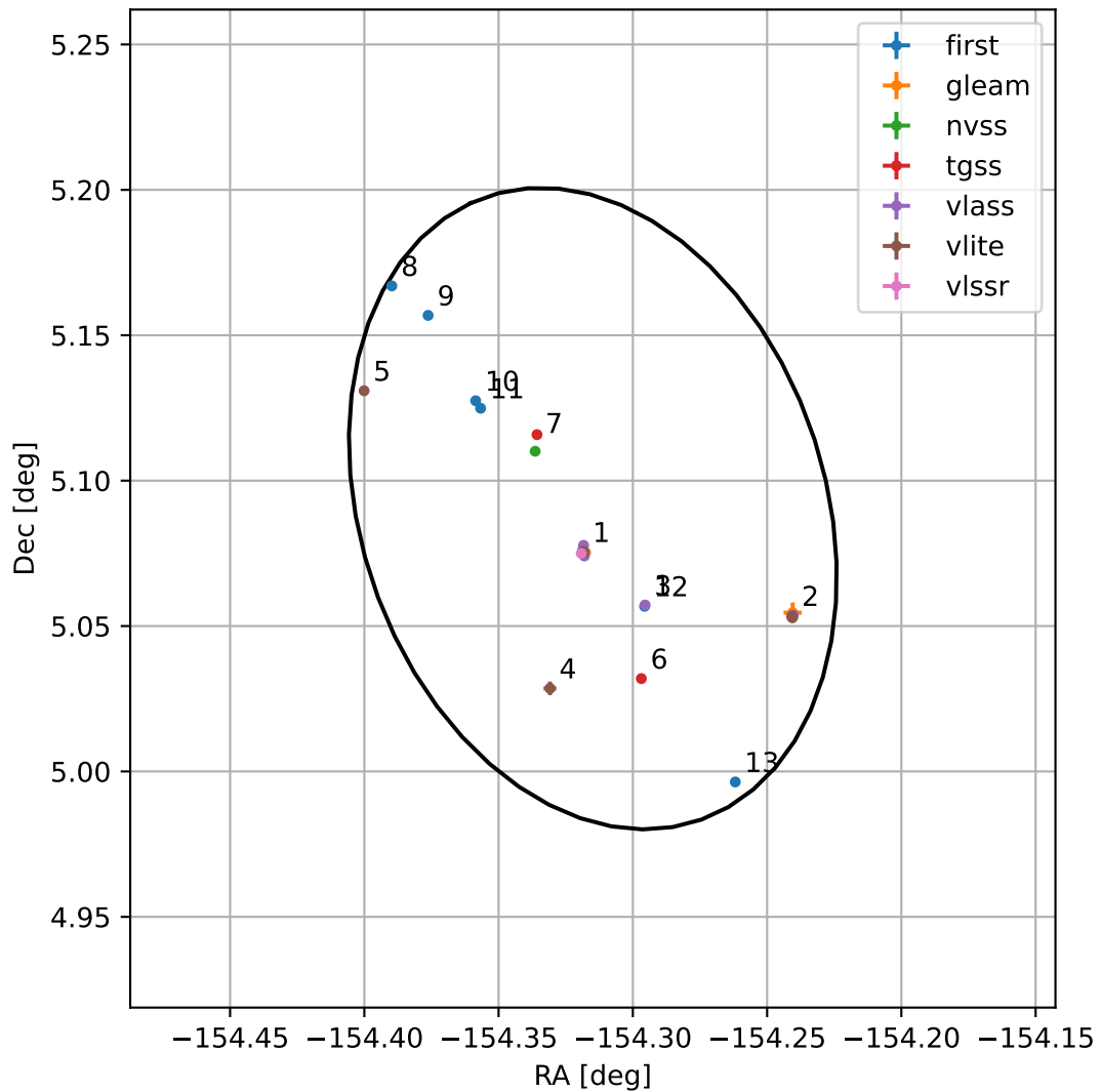
4FGL J1342.7+0505
