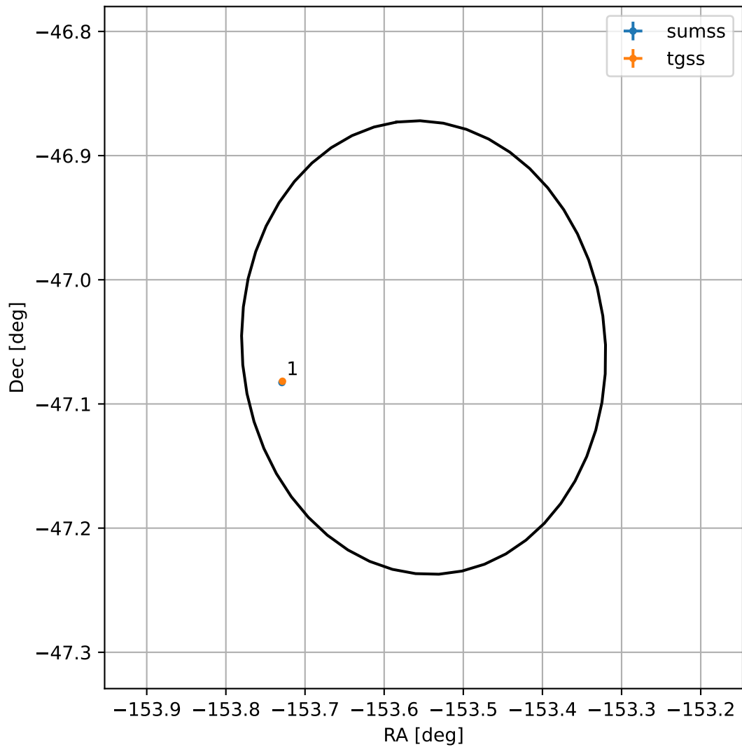
4FGL J1345.7-4703
