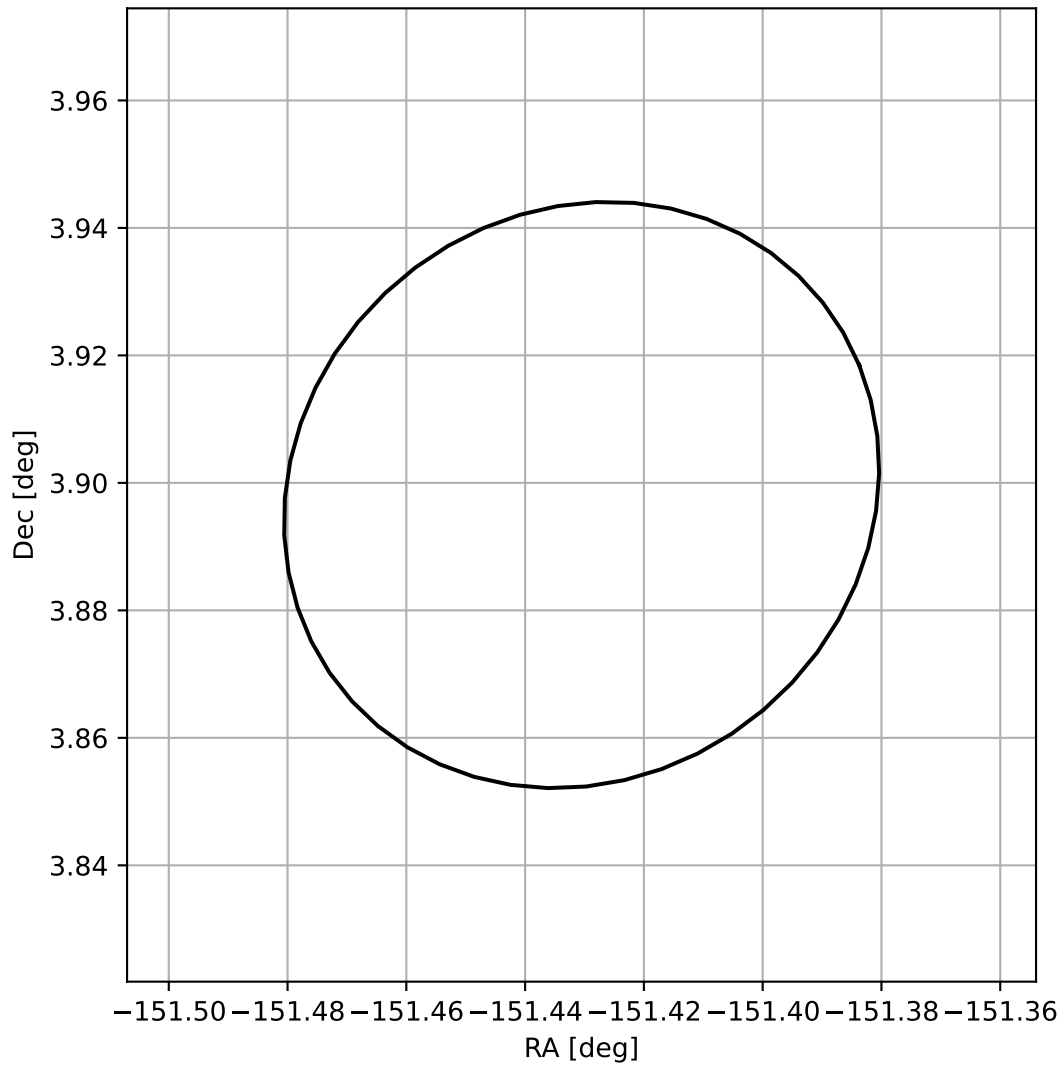
4FGL J1354.2+0353
