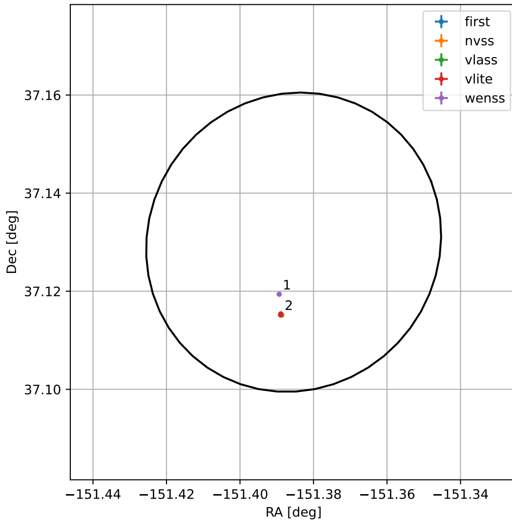
4FGL J1354.4+3707
