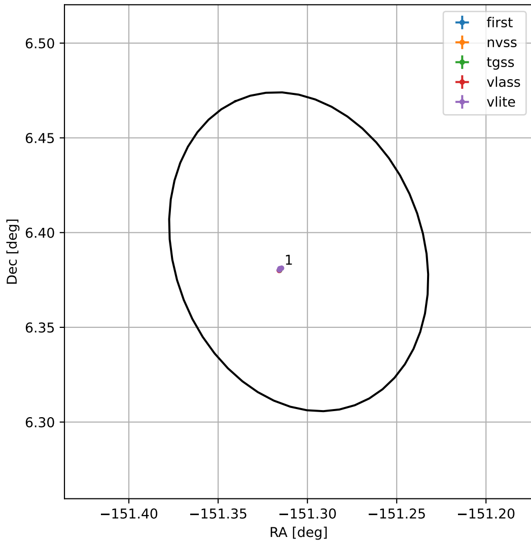
4FGL J1354.7+0623
