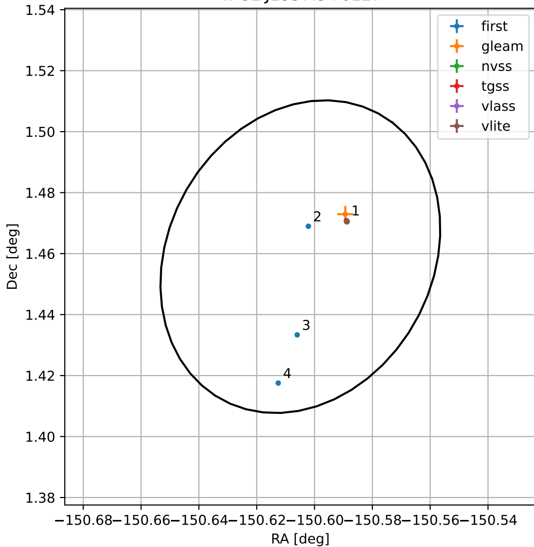
4FGL J1357.5+0127
