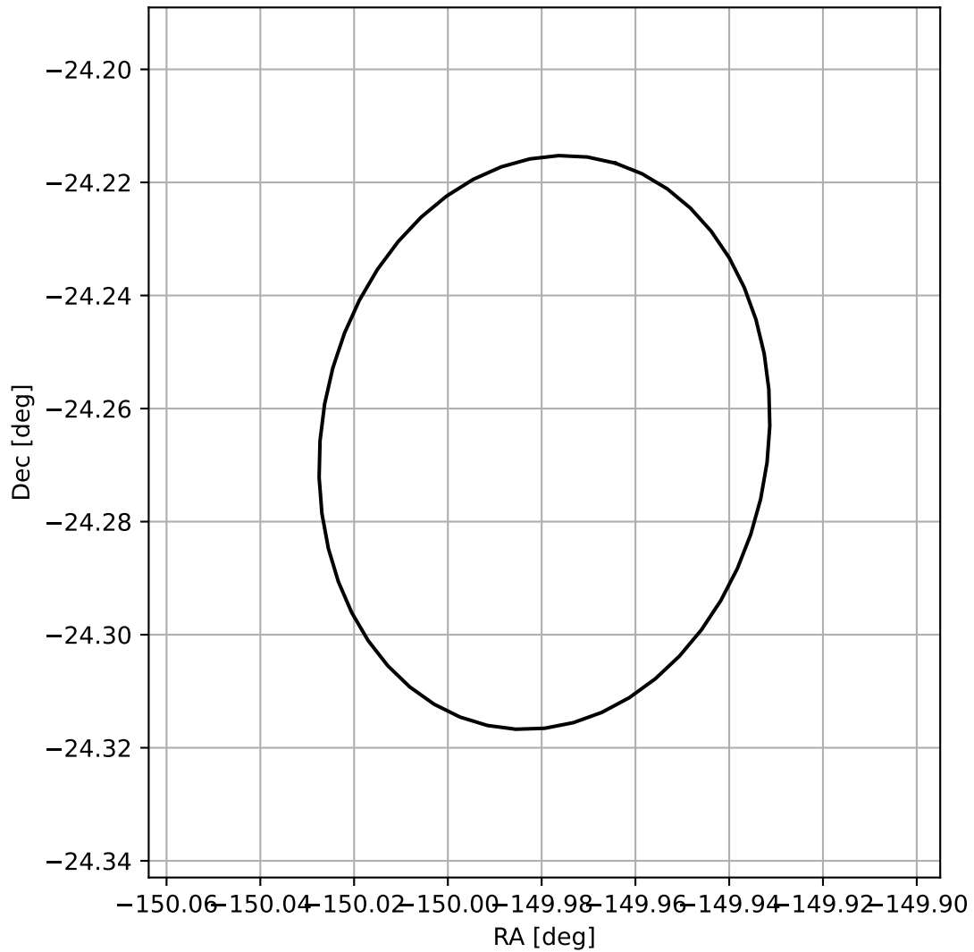
4FGL J1400.0-2415
