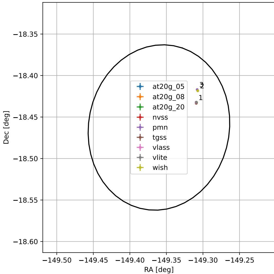
4FGL J1402.5-1827
