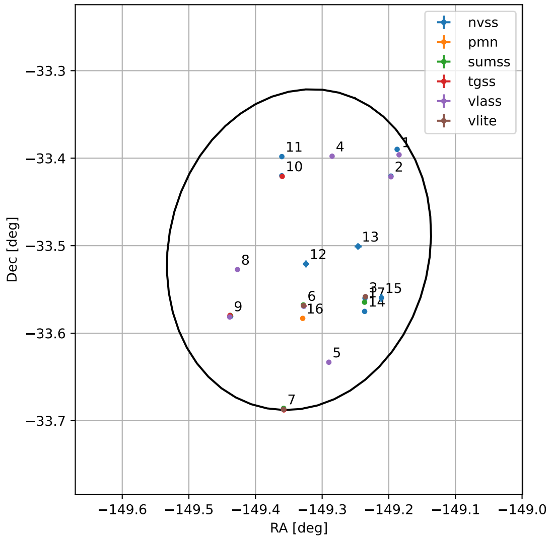
4FGL J1402.6-3330
